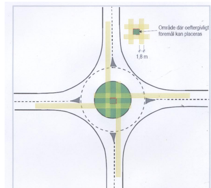
FIGUR 7-127 Område där oeftergivliga föremål kan placeras vid \geq 50 km/h
