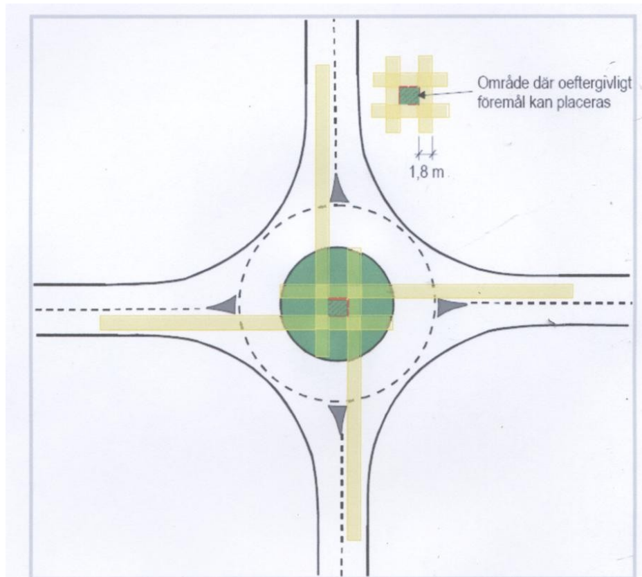
FIGUR 7-127 Område där oefftergivliga föremål kan placeras vid \geq 50 km/h
